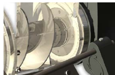
Separasjon mellom hus og transmisjonsenhet
