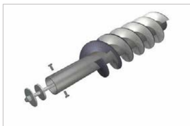
Enkel montering av skruer og deksel
