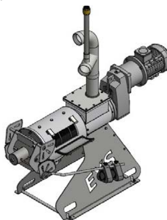
Montering med tilvalgs-utstyr Mounting with Optional Accesories
